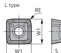
Fig. 3 Centrální destička L type
