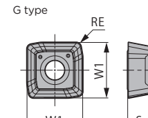
Fig. 4 Centrální destička G type
